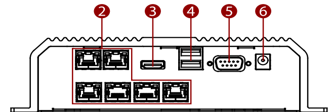
② LAN ③ HDMI ④ USB Type-A ⑤ COM ⑥ Power Input
